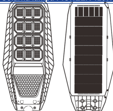
Solárna lampa PIONEER 120W
