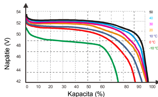
Křivka vybíjení při různých teplotách (0,5 °C)
