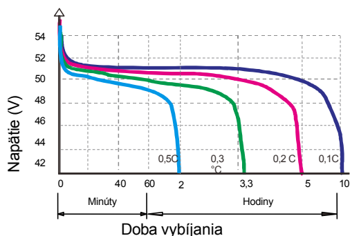
Vybíjecí charakteristiky (25 °C)
