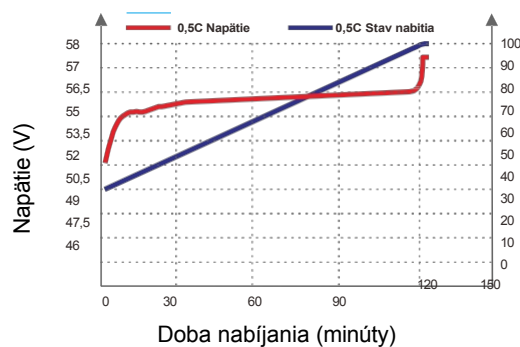
Křivka stavu nabití (0,5 C, 25 °C)
