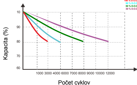
Různé DOD Životnost' vybíjecího cyklu Krivka 0,2C 25 °C
