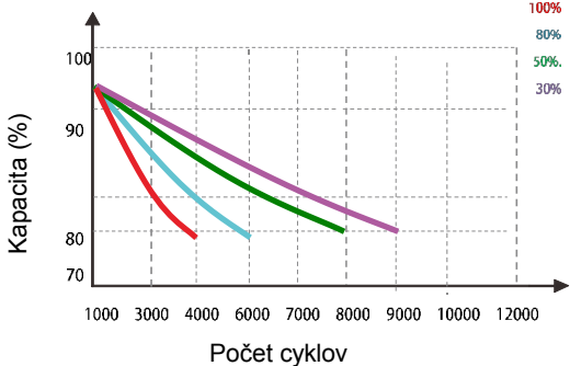
Rôzne DOD Životnosť vybíjacieho cyklu Krivka 0,2C 25 °C
