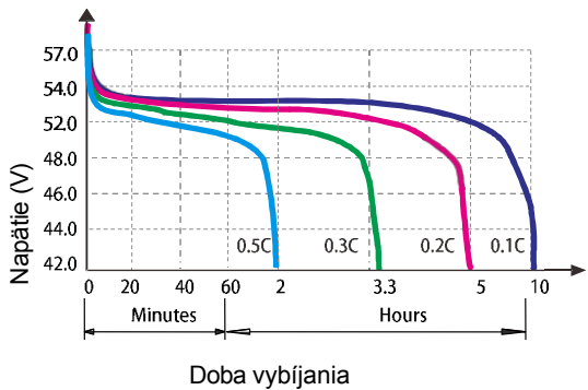
Vlastnosti vybíjania (25 °C)
