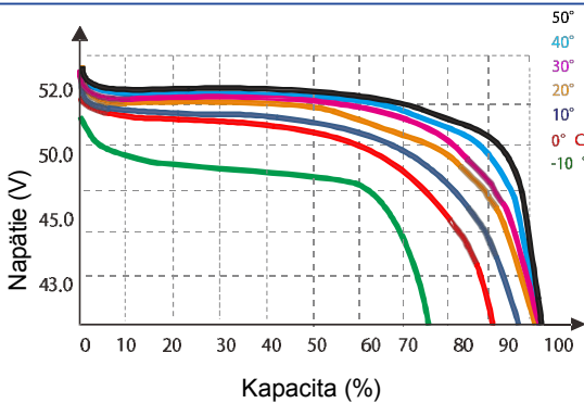
Krivka vybíjania pri rôznych teplotách (0,5 C)
