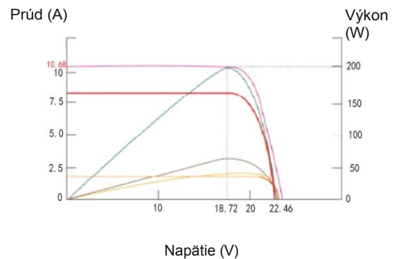
Prúdovo-napät'ové charakteristiky
