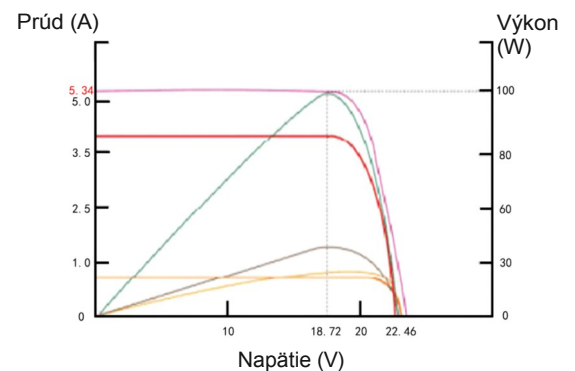
Prúdovo-napät'ové charakteristiky
